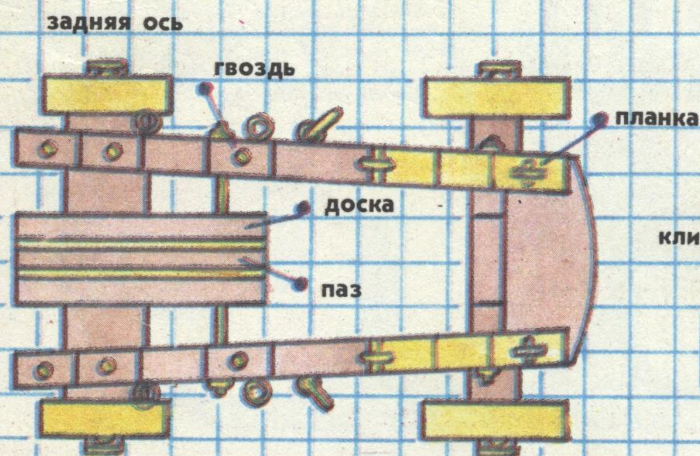
вид сверху (без ствола)
